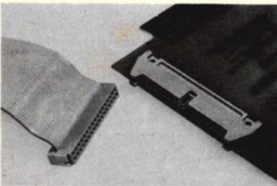
Fig. 1. Op deze manier wordt het zelfstrippende U-contact door de platte kabel geperst, waarna een uitstekende verbinding tussen kabelader tot stand komt. De afb. rechtsboven geeft een zgn. Delta-connector met behuizing voor deze techniek. Links een kabelconnector, die in een printconnector schuift en rechts het handpersje, waarmee alle typen connectoren aan de kabels worden bevestigd.
